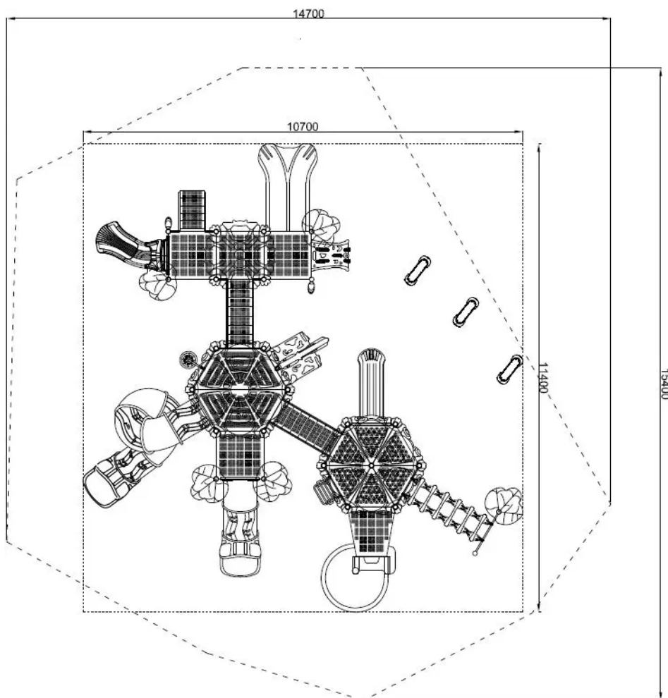
Zał. 1 Wymiary urządzenia
