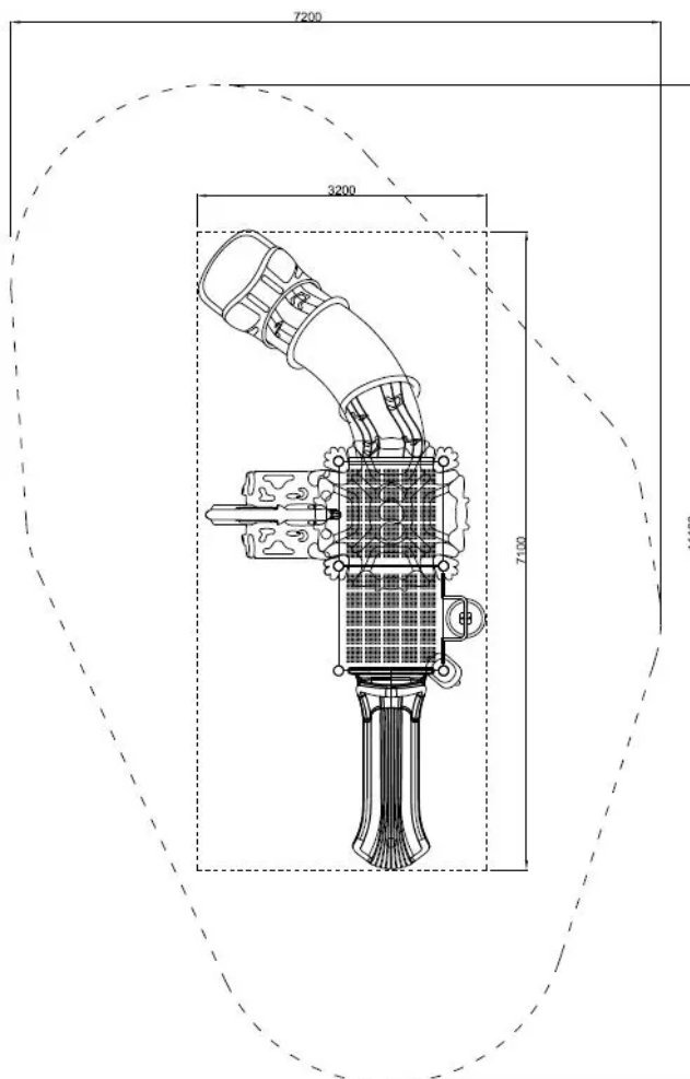
Rys. 1. Wymiary urządzenia i strefy bezpieczeństwa
