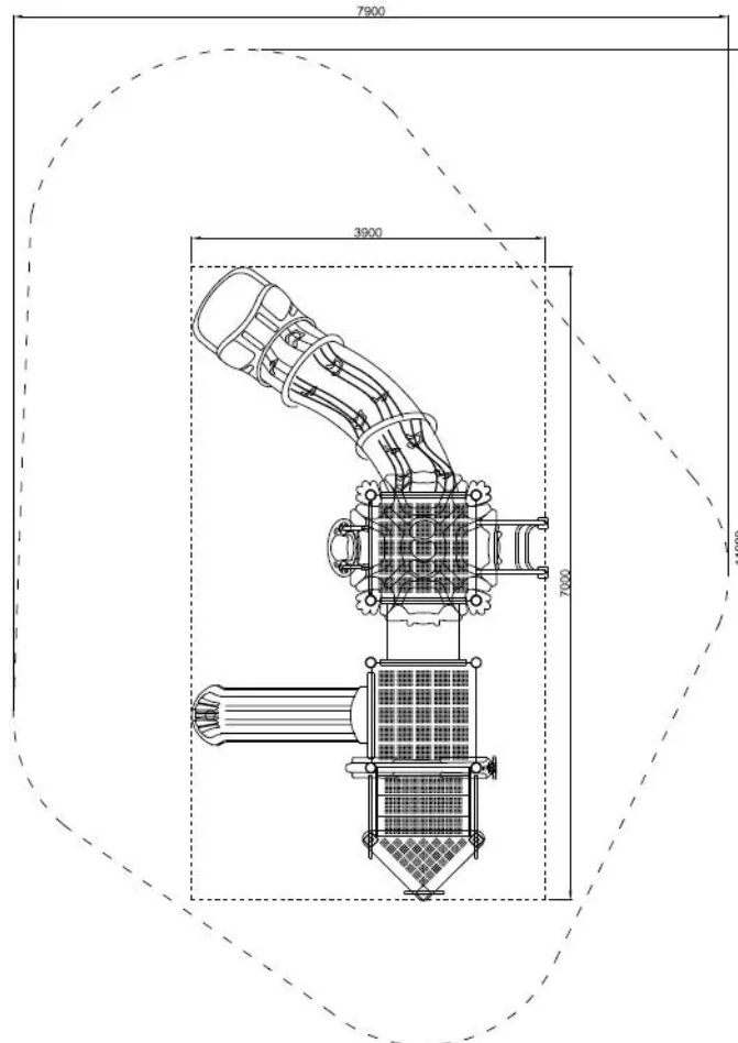
Rys. 1. Wymiary urządzenia i strefy bezpieczeństwa
