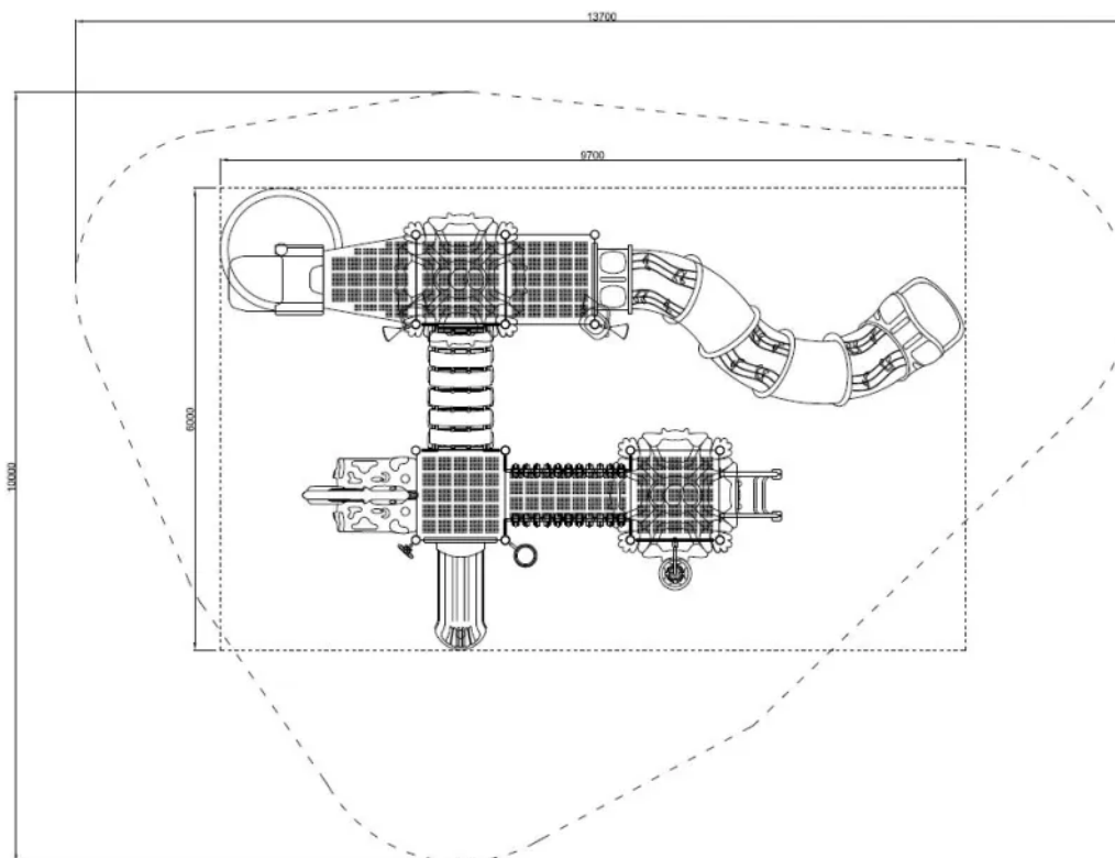
Rys. 1. Wymiary urządzenia i strefy bezpieczeństwa
