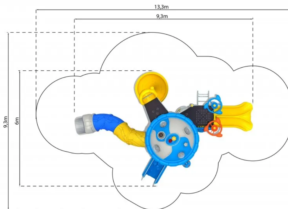
Rys. 1. Wymiary urządzenia i strefy bezpieczeństwa
