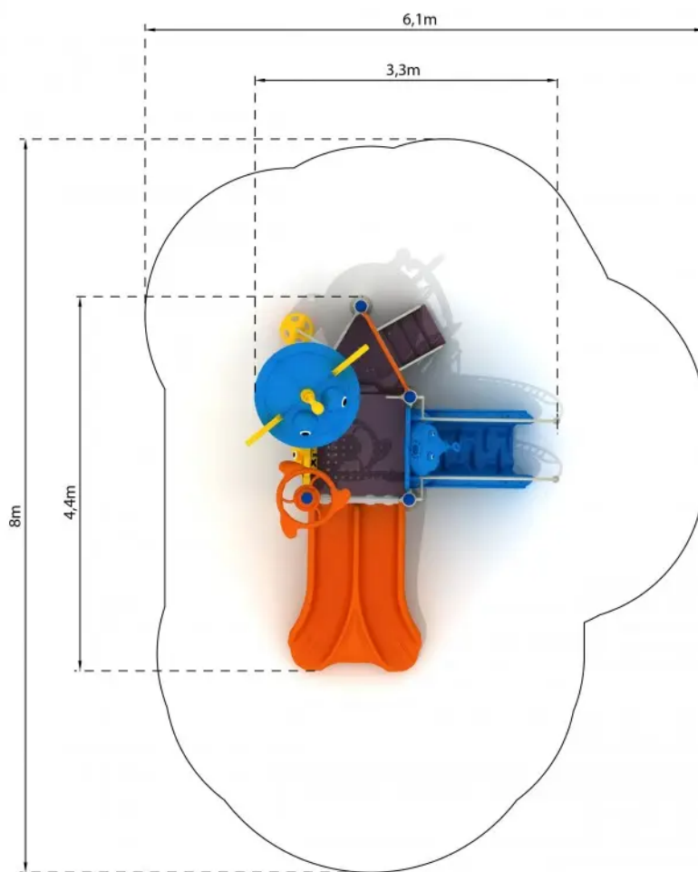
Rys. 1. Wymiary urządzenia i strefy bezpieczeństwa
