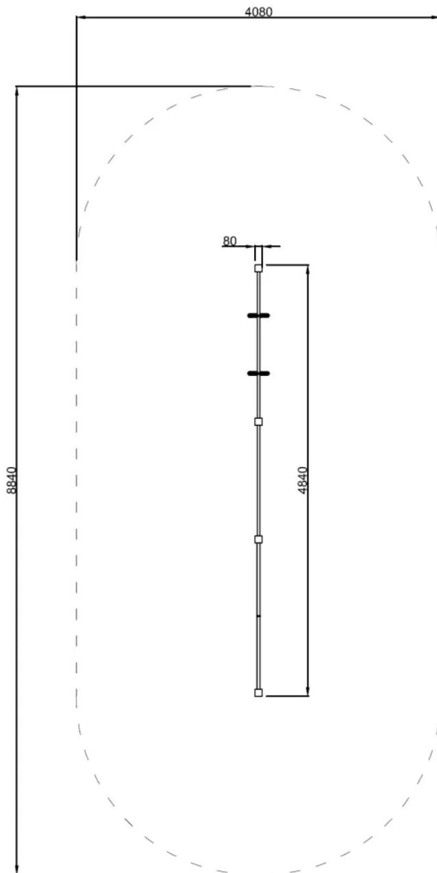
Rys. 1. Wymiary urządzenia i strefy bezpieczeństwa
