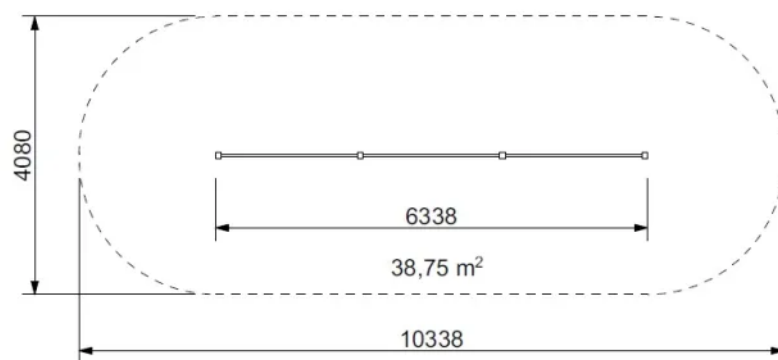
Rys. 1. Wymiary urządzenia i strefy bezpieczeństwa
