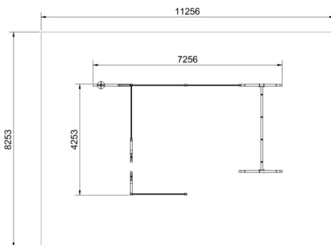
Rys. 1. Wymiary urządzenia i strefy bezpieczeństwa
