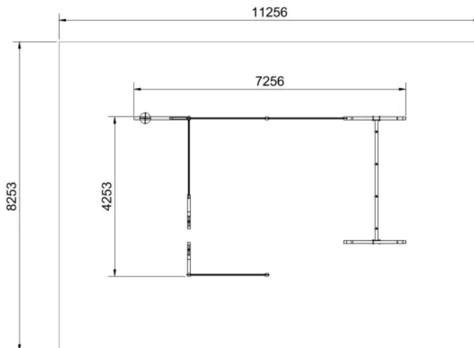
Rys. 1. Wymiary urządzenia i strefy bezpieczeństwa
