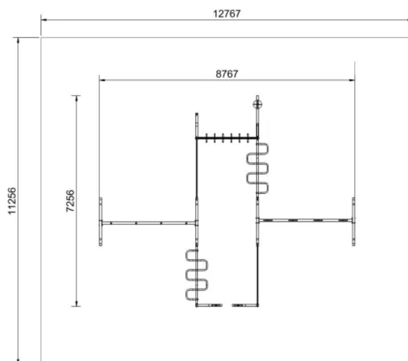
Rys. 1. Wymiary urządzenia i strefy bezpieczeństwa
