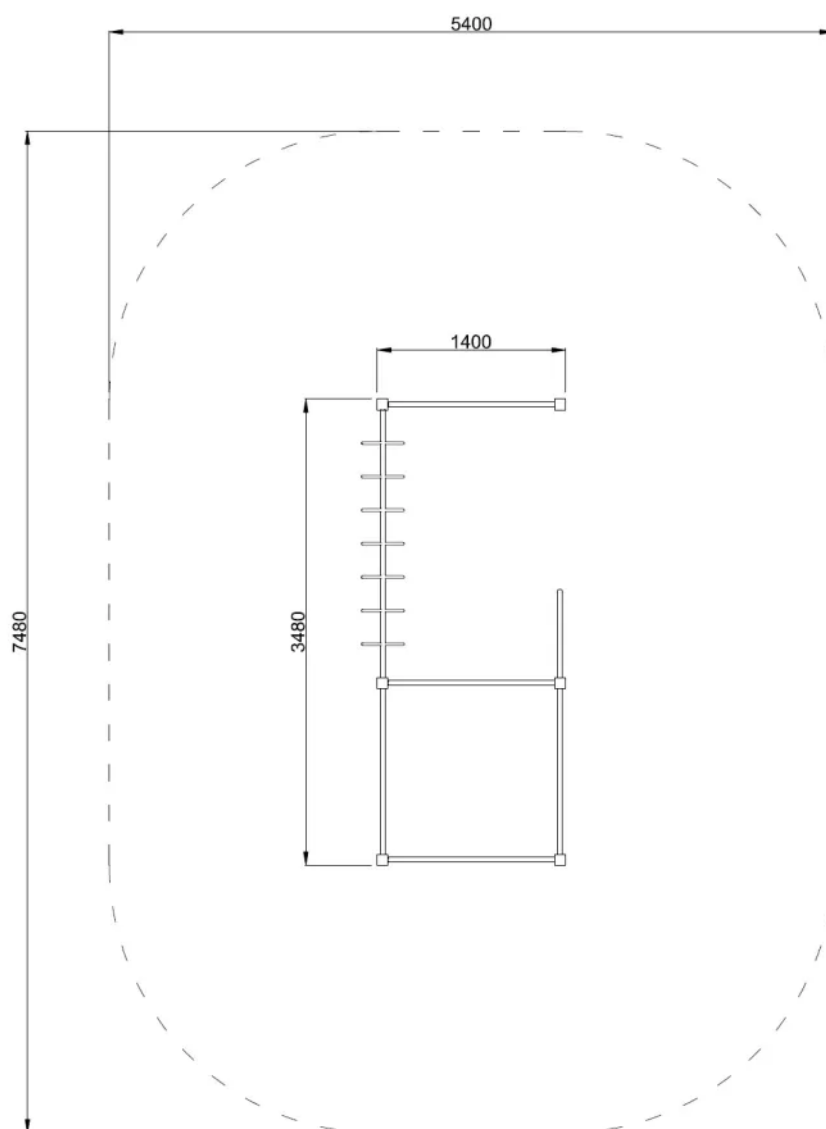
Rys. 1. Wymiary urządzenia i strefy bezpieczeństwa
