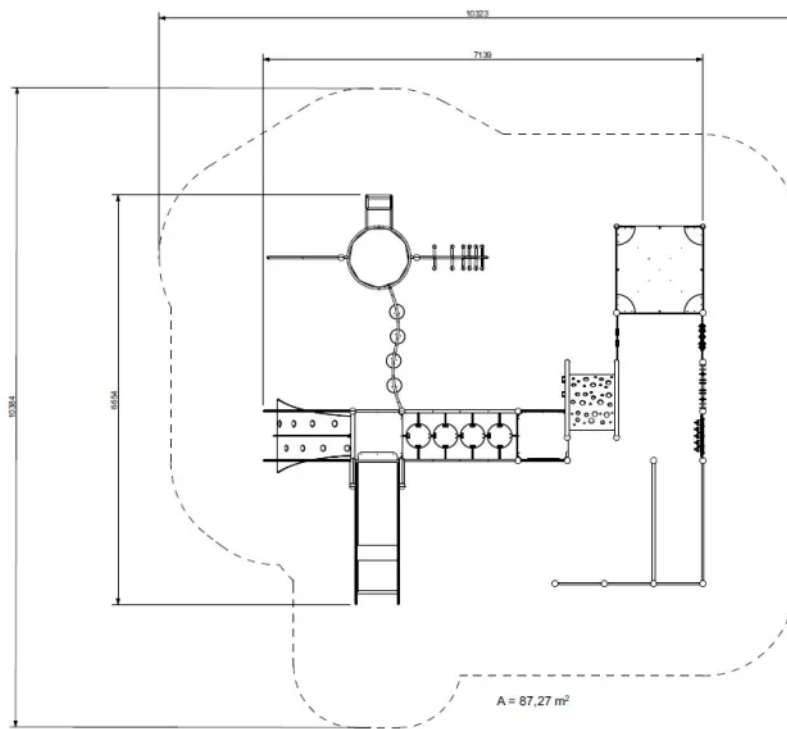
Rys. 1. Wymiary urządzenia i strefy bezpieczeństwa
