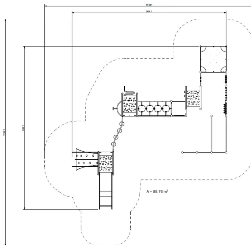
Rys. 1. Wymiary urządzenia i strefy bezpieczeństwa
