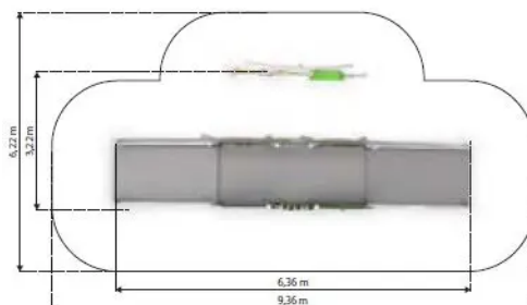
Rys. 1. Wymiary urządzenia i strefy bezpieczeństwa
