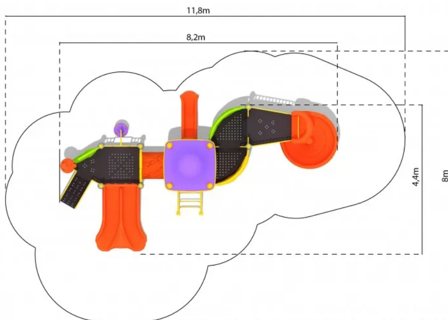
Rys. 1. Wymiary urządzenia i strefy bezpieczeństwa
