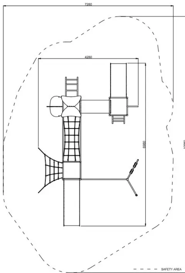
Rys. 1. Wymiary urządzenia i strefy bezpieczeństwa
