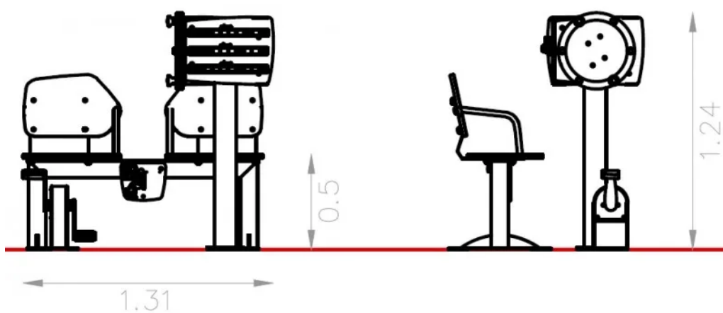
Rys. 1. Wymiary urządzenia i strefy bezpieczeństwa
