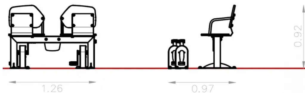
Rys. 1. Wymiary urządzenia
