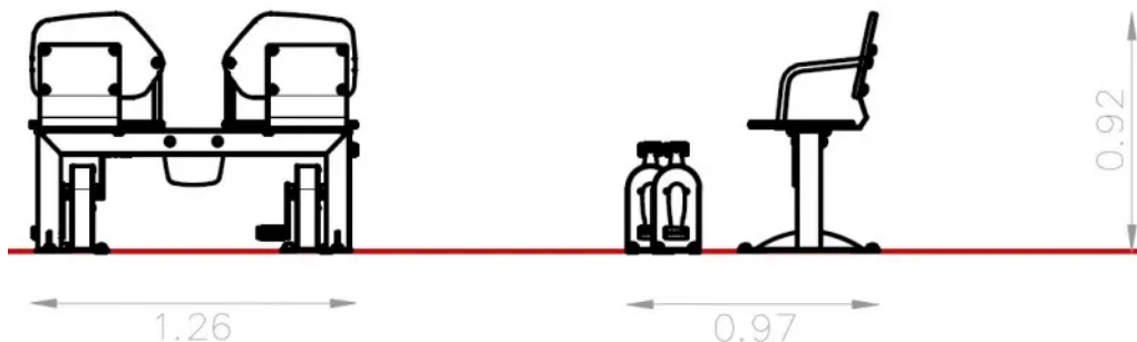
Rys. 1. Wymiary urządzenia
