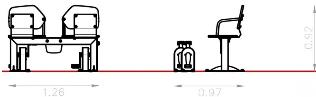
Rys. 1. Wymiary urządzenia
