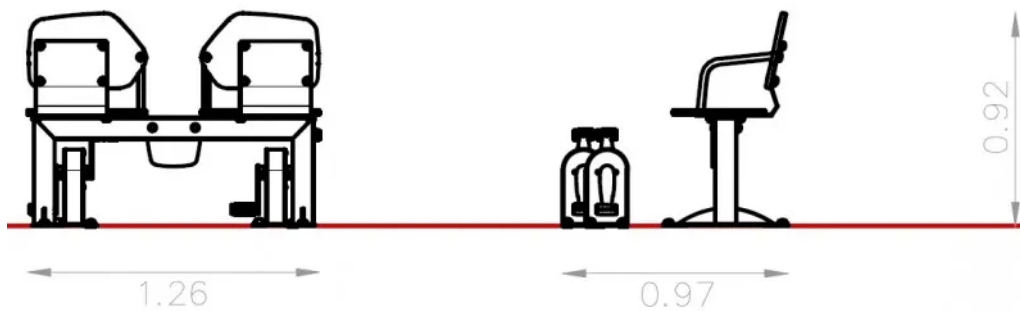
Rys. 1. Wymiary urządzenia
