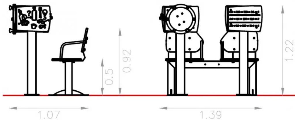
Rys. 1. Wymiary urządzenia i strefy bezpieczeństwa
