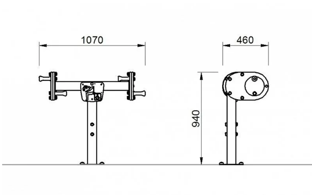
Rys. 1. Wymiary urządzenia i strefy bezpieczeństwa
