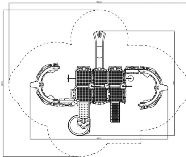
Rys. 1. Wymiary urządzenia i strefy bezpieczeństwa
