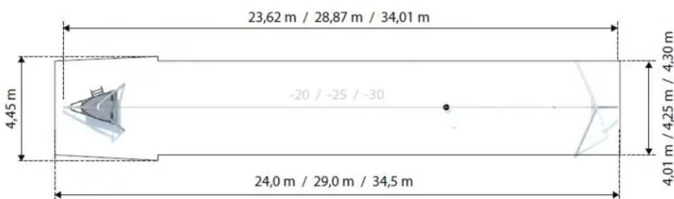
Rys. 1. Wymiary urządzenia i strefy bezpieczeństwa
